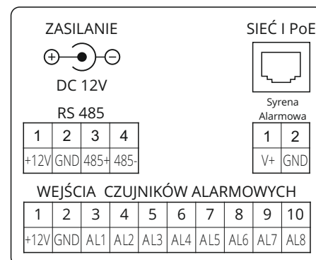
Złącza GR-IS1-WA
