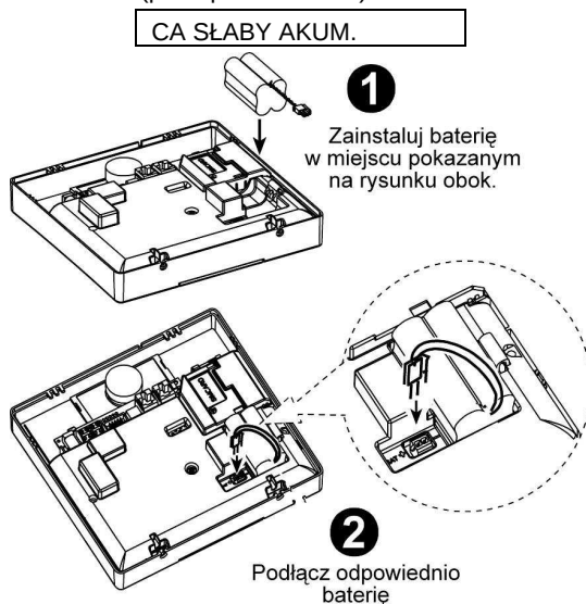
Rysunek 10. Wymiana akumulatorów
