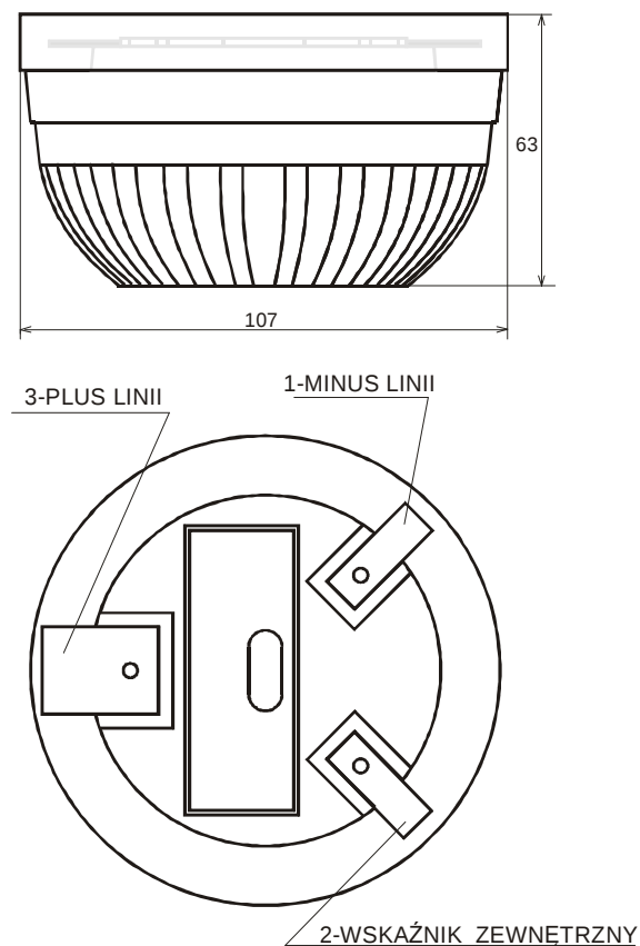
Rys. 2 Wymiary czujki OSD23
