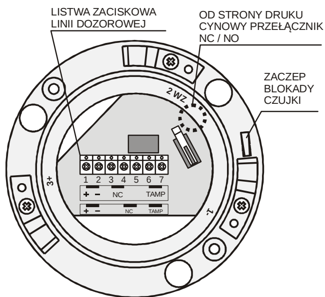
Rys. 4 Gniazdo GNW 12 (GNW24)
