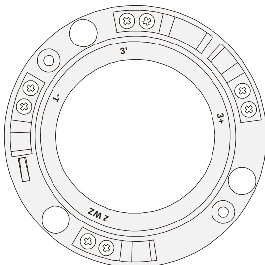
Rys. 3 Gniazdo GNP18
