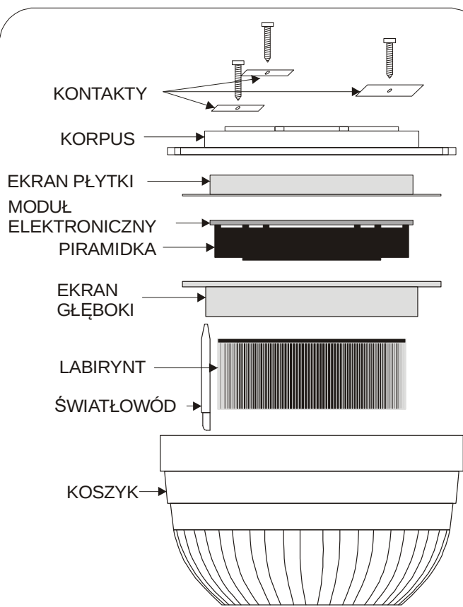
Rys. 1 Budowa czujki
